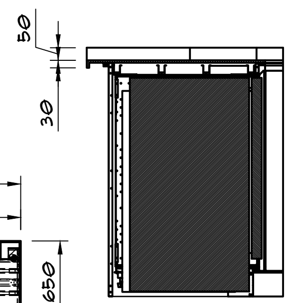
A-A (1:15)
